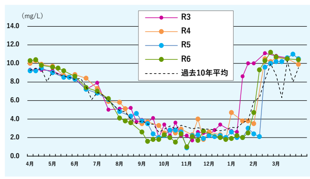
図6 今津沖中央での底層溶存酸素量の経月変動
