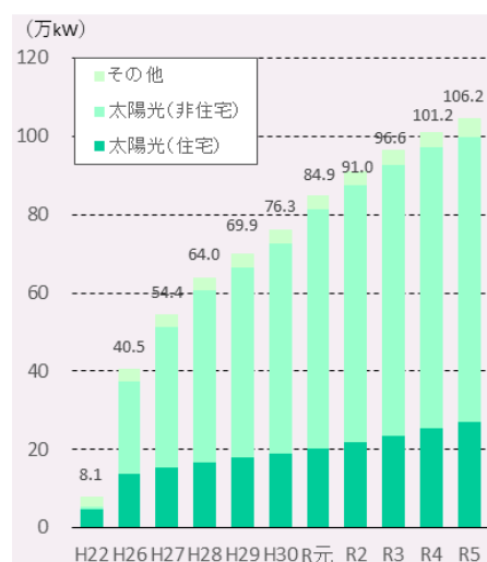
図4 再生可能エネルギー導入量
